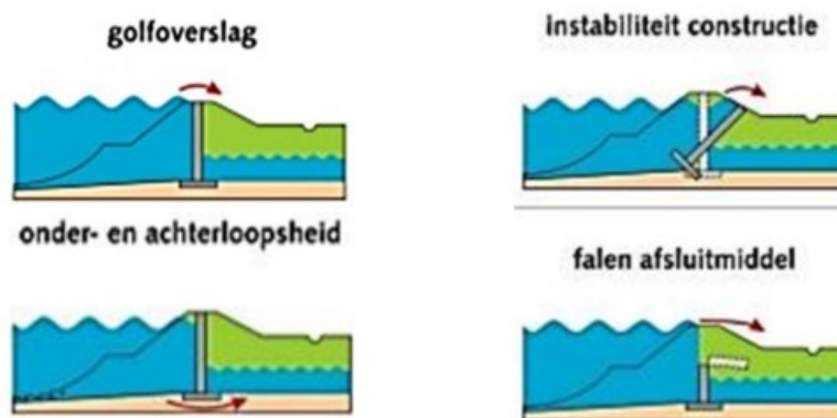
Afbeelding 3.4 Faalmechanismen Katerveercomplex
